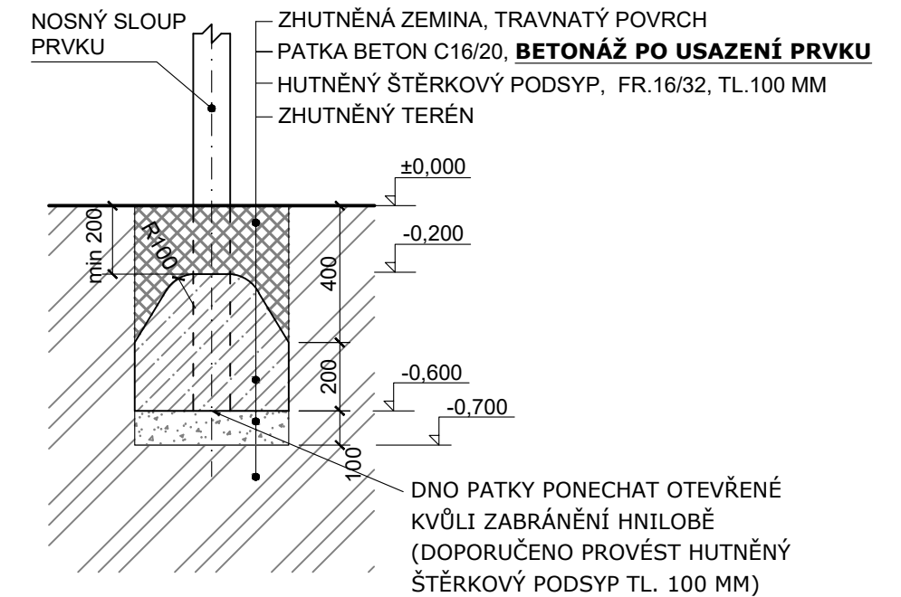
ŘEZ PATKOU
